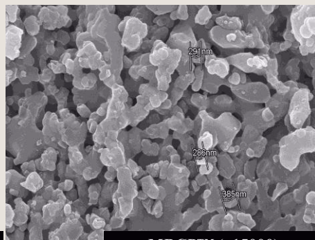
MBCP™ (x15000)
