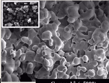
Cerasorb® (x5000)
